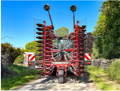
Kverneland barra di semina f-drill CB F trasporto sicuro su strada con ruota di supporto
