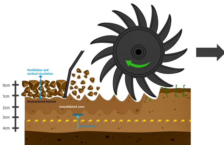
Koncept Helios s konštrukciou hviezdicových kolies s rotačným pohonom
