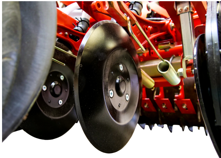
Kverneland f-drill CB F nová výsevná radlička CX-II bez prítlačného kolieska
