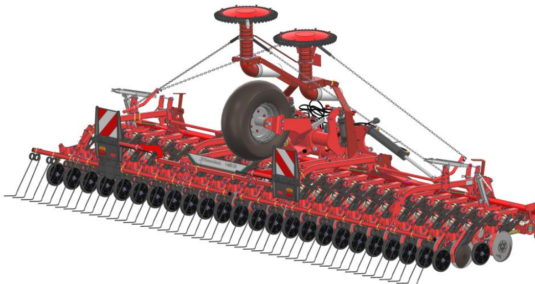
Kverneland f-drill CB F, składana szyna redlic z dwoma głowicami dystrybucyjnymi do systemu podwójnej aplikacji
